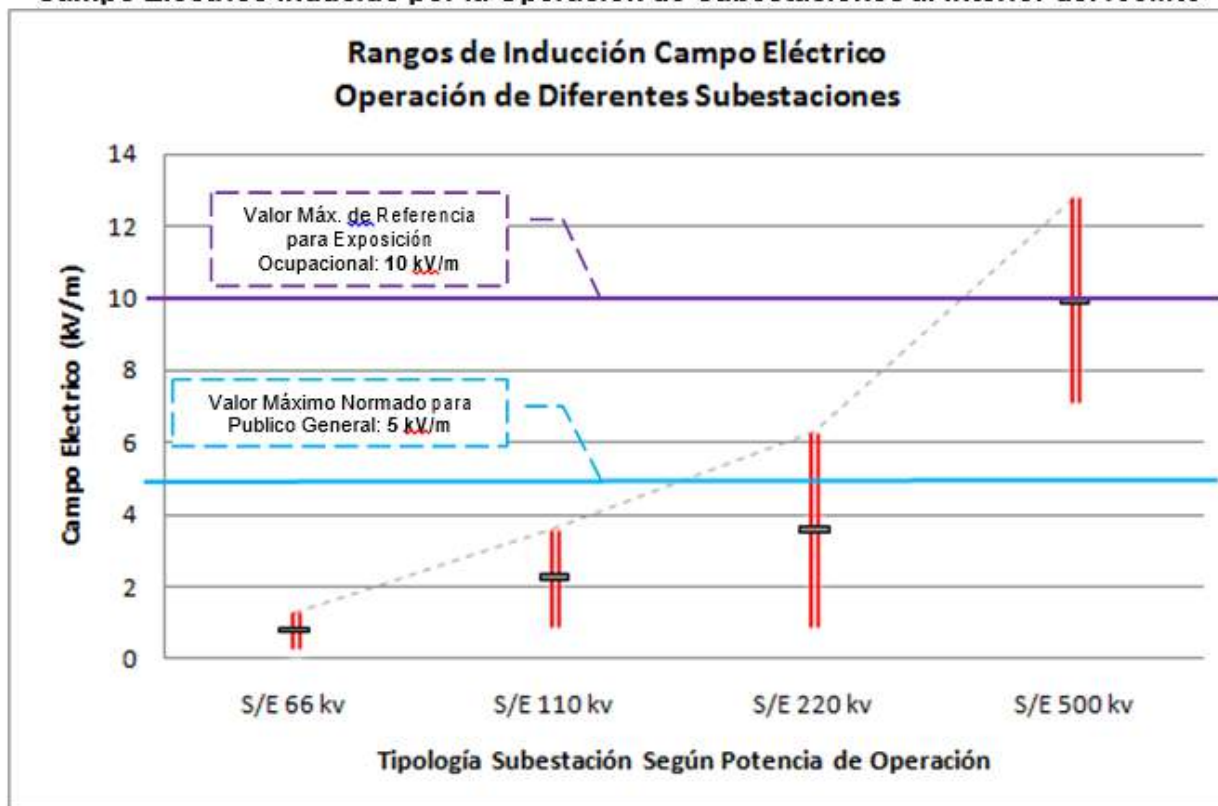
Campo Eléctrico Inducido por la Operación de Subestaciones al interior del recinto
