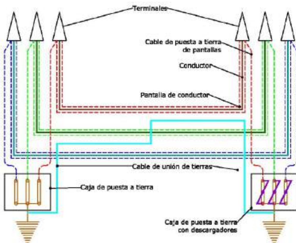
CONEXIÓN TIPO "SINGLE-POINT"
