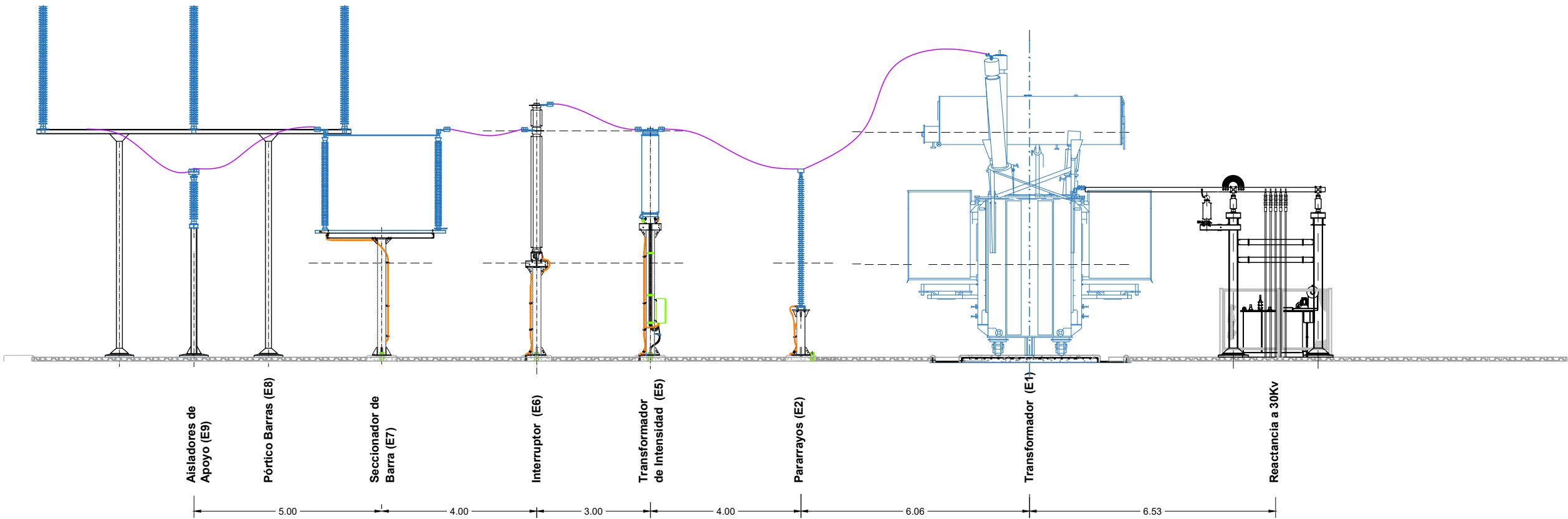
Sección C-C
