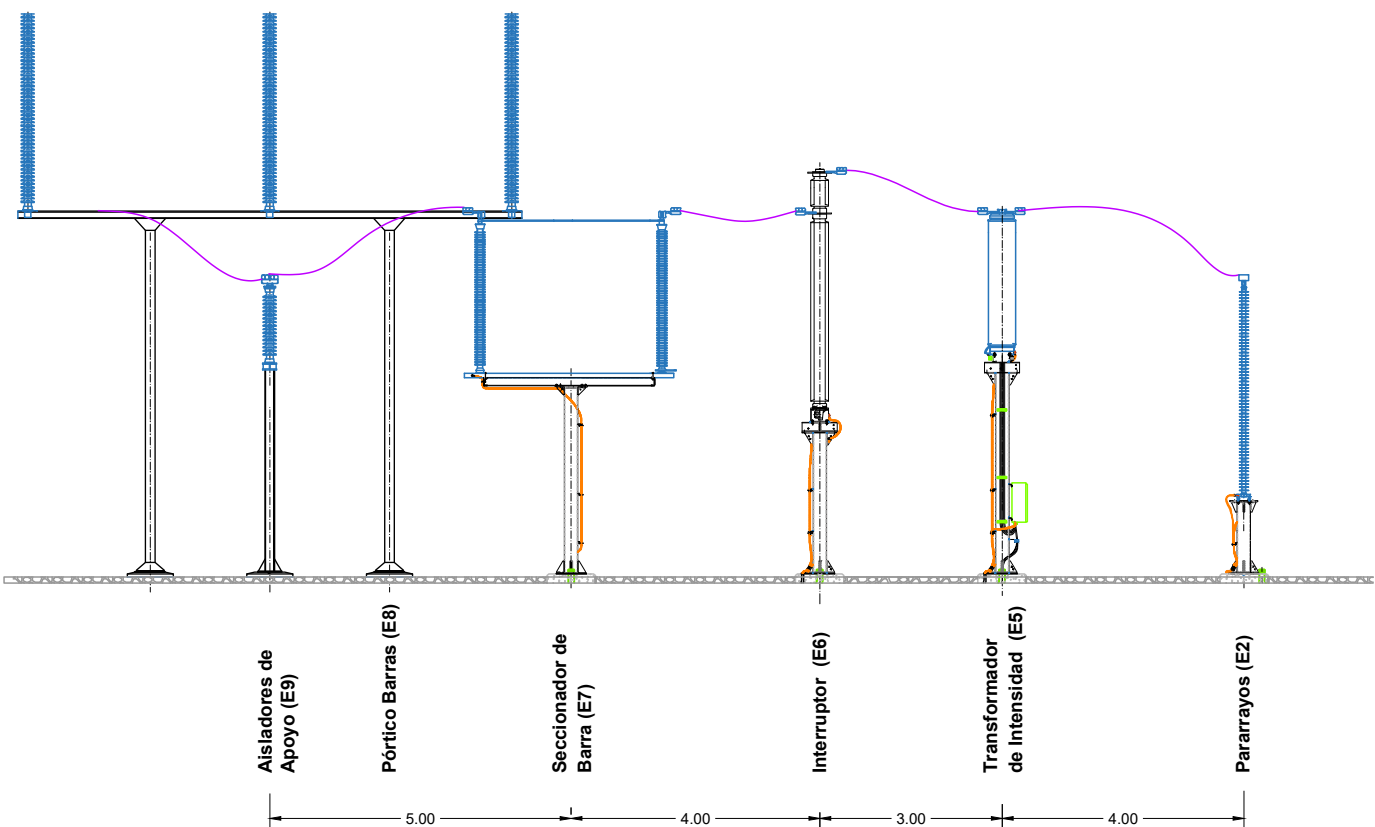
Sección B-B
